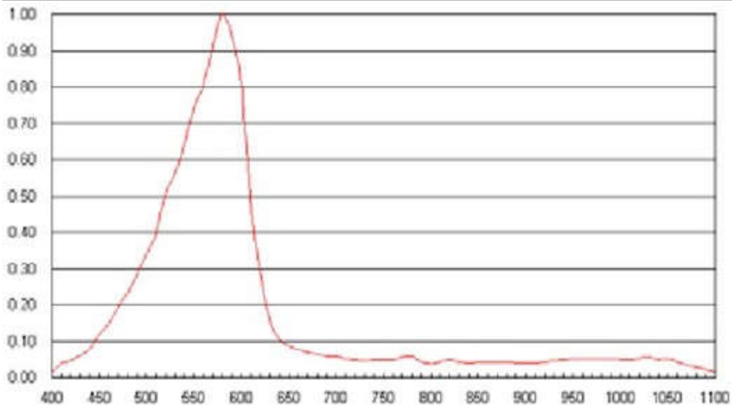
光谱响应曲线
